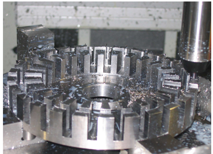
4 assig frezen van een breeschroef
