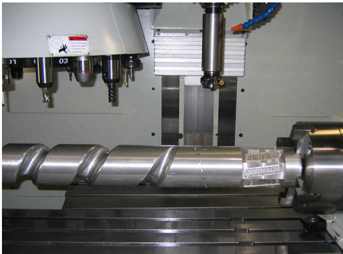
schroeven frezen met oplopende speed
